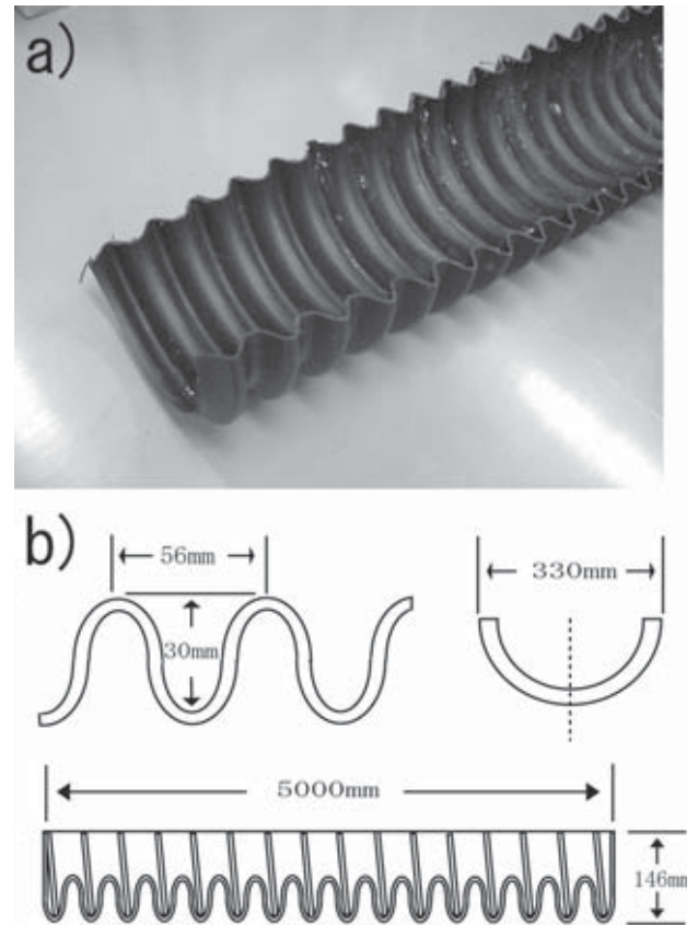
図2 簡易魚道の素材として用いたコルゲート管の規格。 a) コルゲート管の写真、b) コルゲート管の規格
