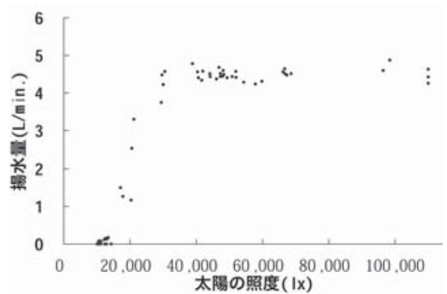
図5 太陽の照度とポンプの揚水量の関係、ソーラーパネルによる太陽光発電によって稼働させたポンプの揚水量を示す。ポンプには13mのホースを接続し、揚程は約2mである。揚水量は照度10,500lxで0.07L/min.、約40,000lxを前後に4～5L/min.で安定した。
