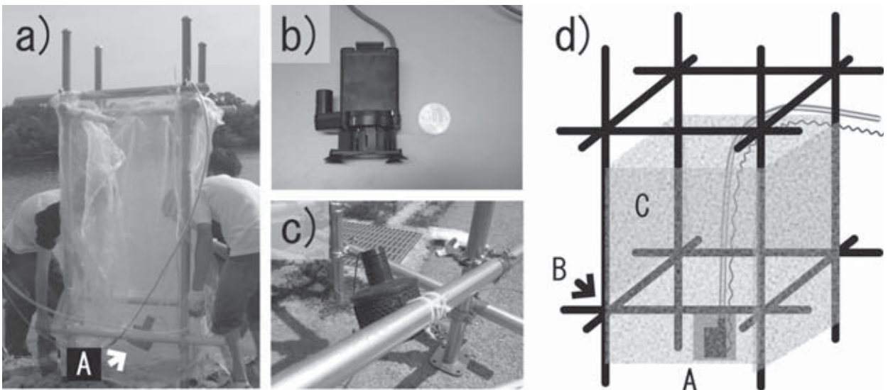
図4 ポンプの設置台. a) 設置台の写真, b) 小型揚水ポンプの写真（500円玉はスケールを示す）, c) ポンプ外付けストレーナーの写真（足場用単管に結束バンドで固定）, d) 設置状況模式図, A: ポンプと外付けストレーナー, B: 足場用単管と自在クランプ, C: 防虫ネットを示す
