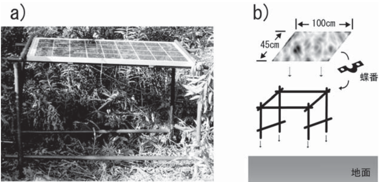
図3 ソーラーパネルの設置台. a) 設置台の写真, b) 設置状況模式図
