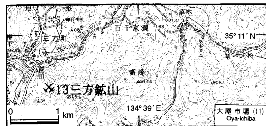
第6図. 三方鉱山の位置図。国土地理院発行5万分の1地形図「大屋市場」を使用。
