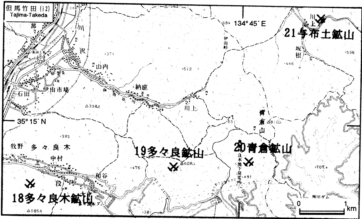
第9図. 多々良木鉱山・多々良鉱山・青倉鉱山・与布土鉱山の位置図・国土地理院発行5万分の1地形図「但馬竹田」を使用。
