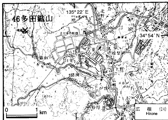
第20図. 多田鉦山の位置図. 国土地理院発行5万分の1地形図「広根」を使用.
