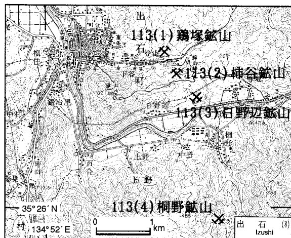
第66図. 鶏塚鉱山・柿谷鉱山・日野辺鉱山・桐野鉱山の位置図. 国土地理院発行5万分の1地形図「出石」を使用.
