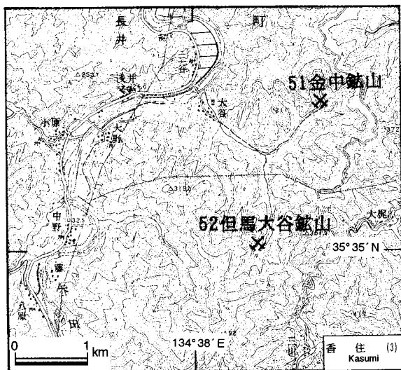
第25図. 金中鉾山・但馬大谷鉾山の位置図. 国土地理院発行5万分の1地形図「香住」を使用。
