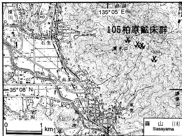
第59図. 柏原鉾床群の位置図. 国土地理院発行 5 万分の 1 地形図「篠山」を使用.
