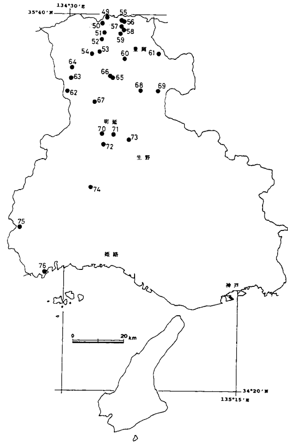
第23図. 兵庫県下の金・銀鉱床の分布. 番号は本文中の鉱山・鉱床の番号に対応する.
