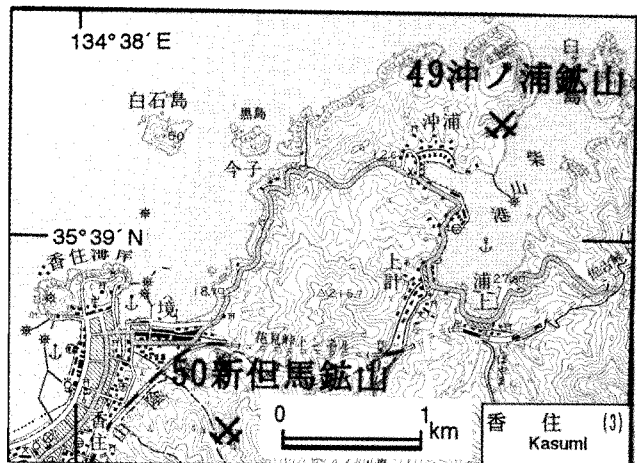
第24図. 沖ノ浦鉱山・新但馬鉱山の位置図. 国土地理院発行5万分の1地形図「香住」を使用.
