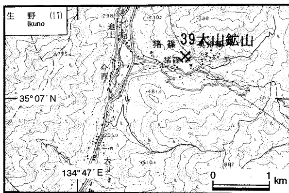
第16図. 大山鉱山の位置図。国土地理院発行5万分の1地形図「生野」を使用。
