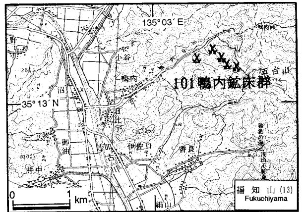
第57図. 鴨内鉱床群の位置図. 国土地理院発行5万分の1地形図「福知山」を使用.
