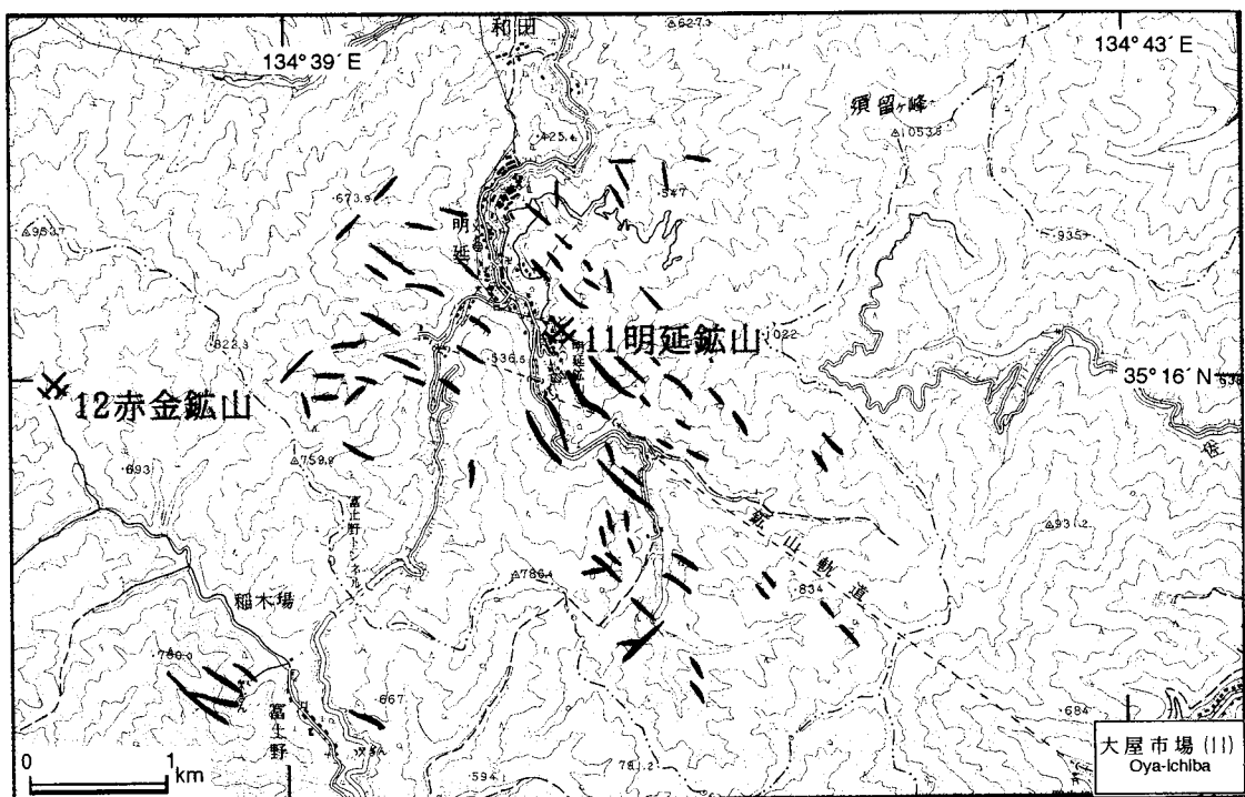
第5図. 明延鉱山・赤金鉱山の位置図. 国土地理院発行5万分の1地形図「大屋市場」を使用。
