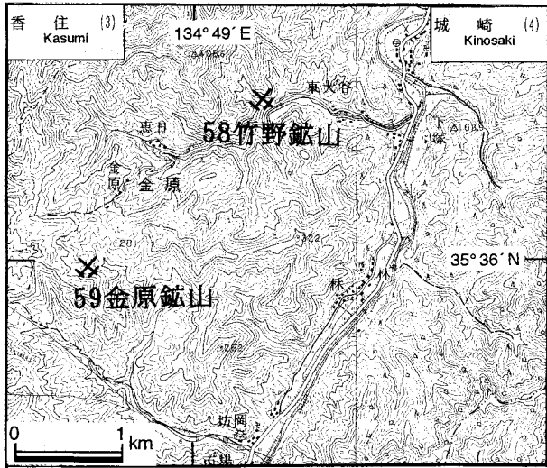
第28図. 竹野鉱山・金原鉱山の位置図. 国土地理院発行5万分の1地形図「香住」「城崎」を使用.
