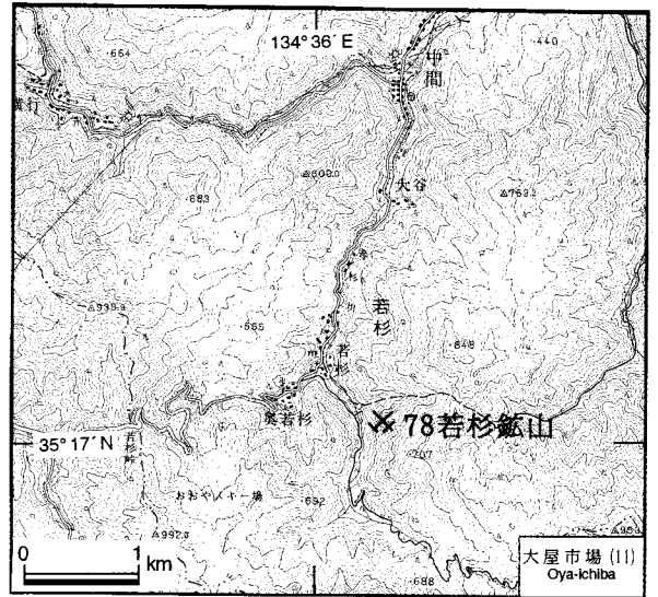
第47図. 若杉鉱山の位置図. 国土地理院発行5万分の1地形図「大屋市場」を使用.
