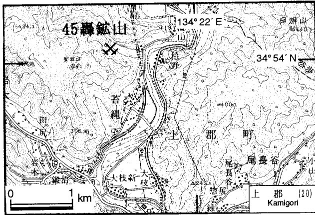
第19図. 轟鉦山の位置図. 国土地理院発行5万分の1地形図「上郡」を使用.
