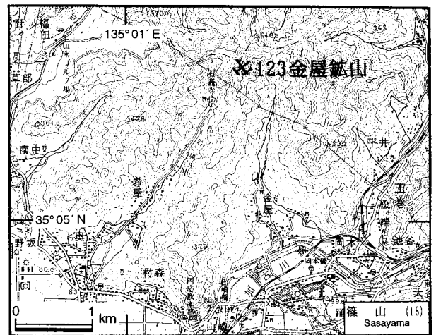
第71図. 金屋鉱山の位置図. 国土地理院発行5万分の1地形図「篠山」を使用.
