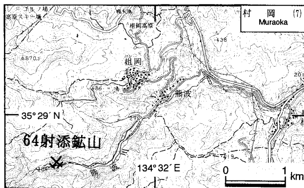
第33図. 射添鉱山の位置図。国土地理院発行5万分の1地形図「村岡」を使用。
