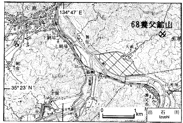
第36図. 養父鉱山の位置図. 国土地理院発行5万分の1地形図「出石」を使用.
