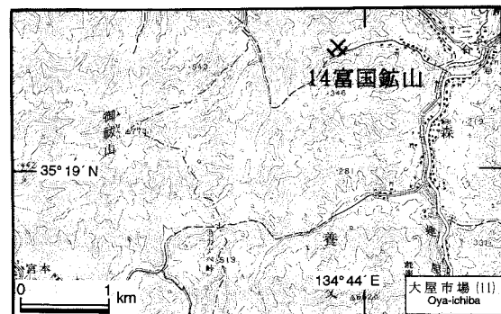
第7図. 富国鉱山の位置図。国土地理院発行5万分の1地形図「大屋市場」を使用。
