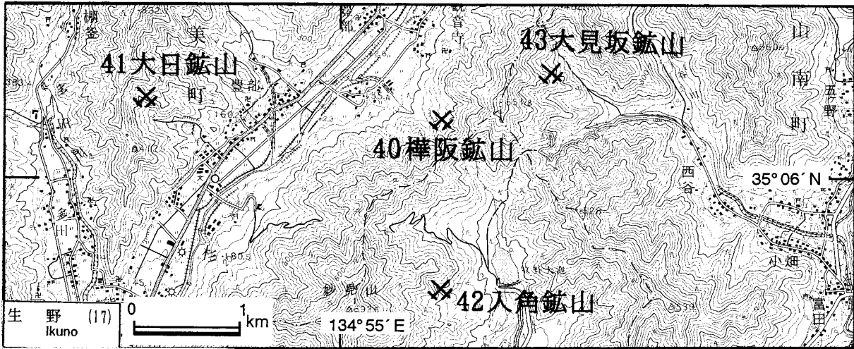
第17図. 樺阪鉱山・大日鉱山・入角鉱山・大見坂鉱山の位置図. 国土地理院発行5万分の1地形図「生野」を使用.
