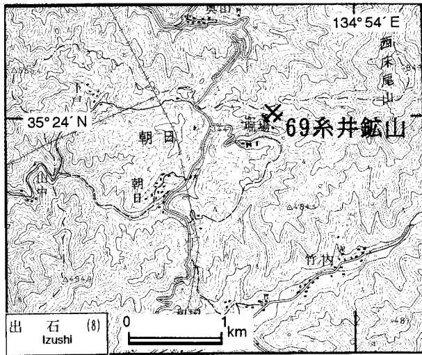
第37図. 糸井鉱山の位置図. 国土地理院発行5万分の1地形図「出石」を使用.
