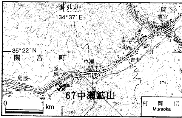
第35図. 中瀬鉱山の位置図. 国土地理院発行5万分の1地形図「村岡」を使用.
