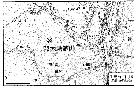
第41図. 大乘鉱山の位置図. 国土地理院発行5万分の1地形図「但馬竹田」を使用.
