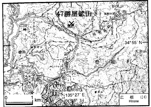
第21図. 勝星鉦山の位置図. 国土地理院発行5万分の1地形図「広根」を使用.
