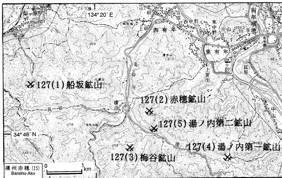
第75図. 船坂鉱山・赤穂鉱山・梅谷鉱山・湯ノ内第一鉱山・湯ノ内第二鉱山の位置図. 国土地理院発行5万分の1地形図「播州赤穂」を使用.
