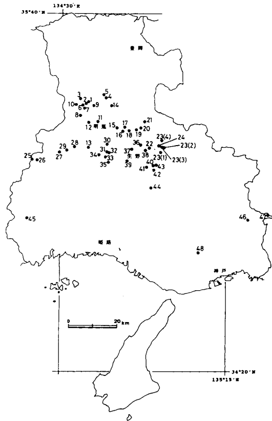
第1図 兵庫県下の多金属鉱床の分布。番号は本文中の鉱山・鉱床の番号に対応する。
