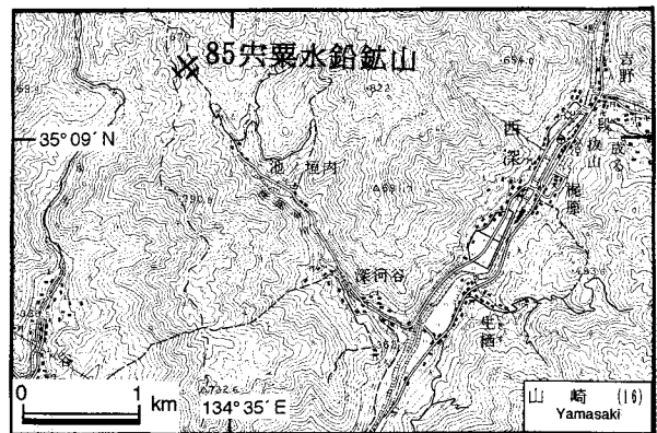
第53図. 穴栗水鉛鉱山の位置図. 国土地理院発行5万分の1地形図「山崎」を使用.
