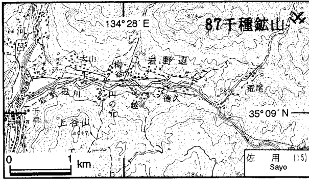
第55図. 千種鉱山の位置図. 国土地理院発行5万分の1地形図「佐用」を使用.
