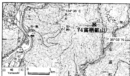
第42図. 富栖鉱山の位置図. 国土地理院発行5万分の1地形図「山崎」を使用.
