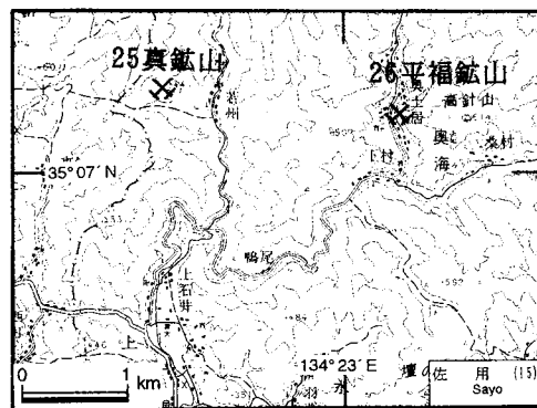
第11図. 真鉱山・平福鉱山の位置図. 国土地理院発行5万分の1地形図「佐用」を使用.
