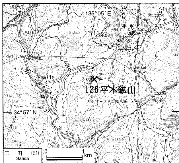
第74図. 平木鉱山の位置図. 国土地理院発行5万分の1地形図「三田」を使用.
