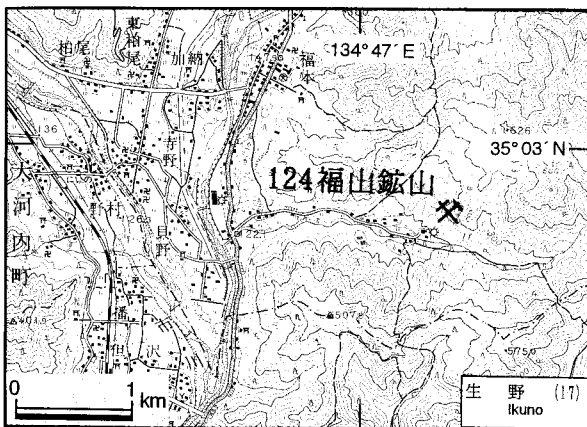
第72図. 福山鉱山の位置図。国土地理院発行5万分の1地形図「生野」を使用。
