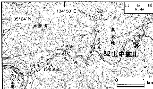
第50図. 山中鉱山の位置図。国土地理院発行5万分の1地形図「出石」を使用。
