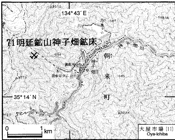
第39図. 明延鉱山神子畑鉱床の位置図. 国土地理院発行5万分の1地形図「大屋市場」を使用.
