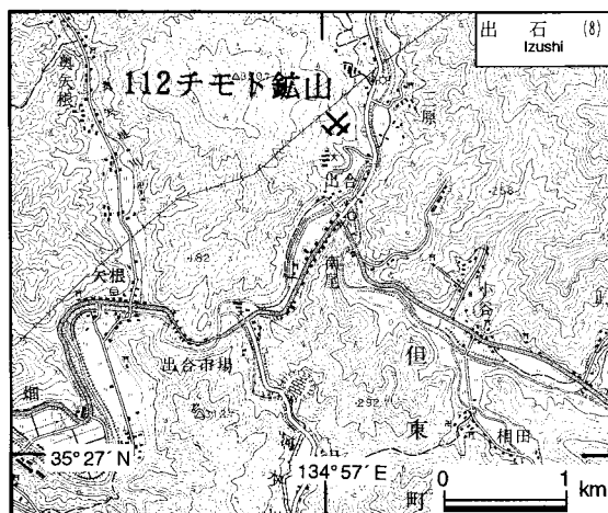
第65図. チモト鉱山の位置図. 国土地理院発行5万分の1地形図「出石」を使用.
