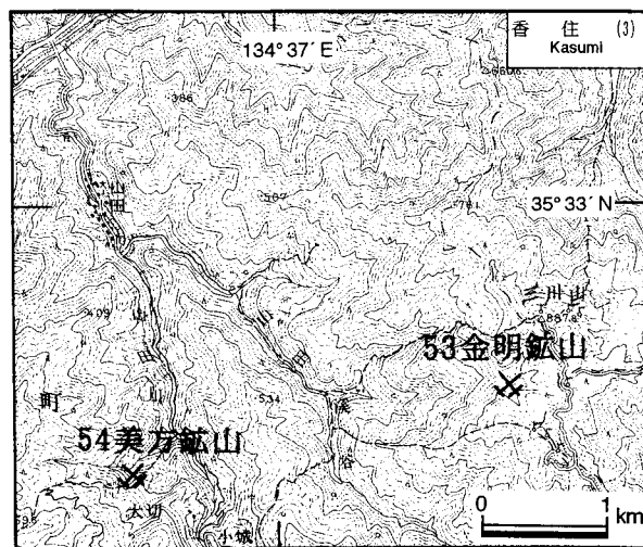
第26図. 金明鉾山・美方鉾山の位置図. 国土地理院発行5万分の1地形図「香住」を使用。
