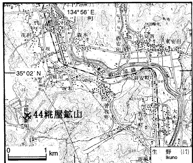
第18図. 糺屋鉱山の位置図. 国土地理院発行5万分の1地形図「生野」を使用.
