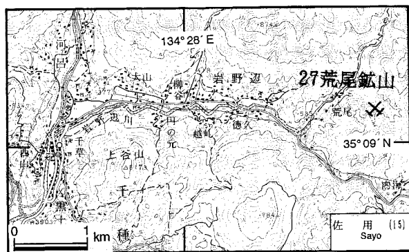
第12図. 荒尾鉱山の位置図. 国土地理院発行5万分の1地形図「佐用」を使用。
