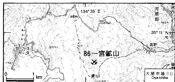
第54図. 一宮鉱山の位置図. 国土地理院発行5万分の1地形図「大屋市場」を使用.
