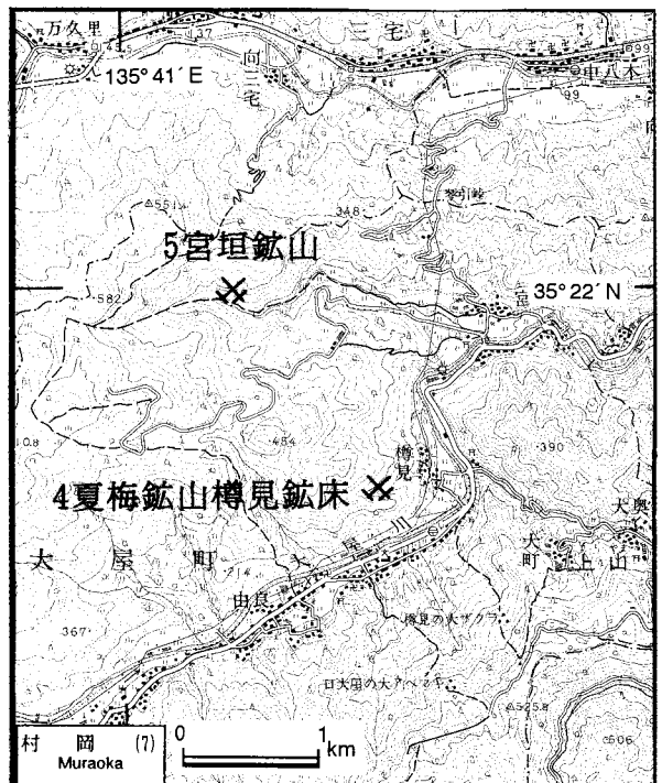
第3図 夏梅樽見鉱山・宮垣鉱山の位置図。国土地理院発行5万分の1地形図「村岡」を使用。
