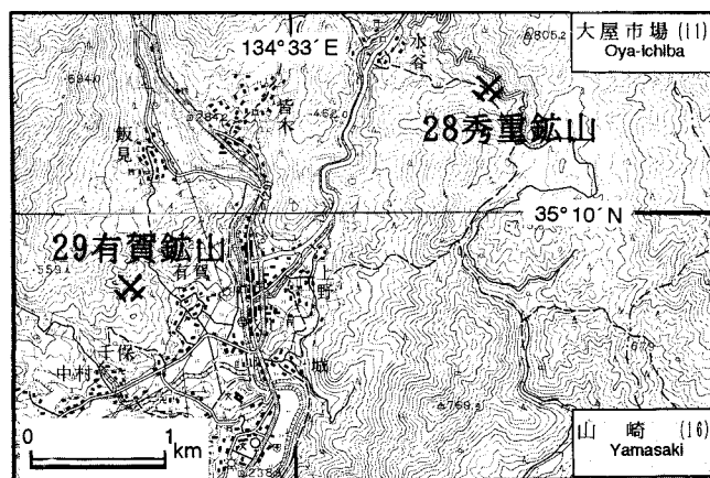
第13図. 秀重鉱山・有賀鉱山の位置図. 国土地理院発行5万分の1地形図「大屋市場」「山崎」を使用。
