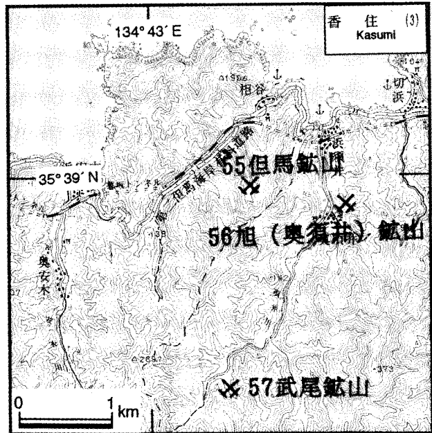
第27図. 但馬鉱山・旭(奥須井)鉱山・武尾鉱山の位置図. 国土地理院発行5万分の1地形図「香住」を使用.
