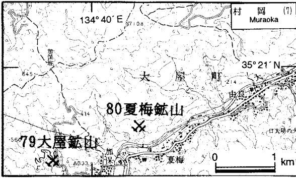
第48図. 夏梅鉱山・大屋鉱山の位置図. 国土地理院発行5万分の1地形図「村岡」を使用.
