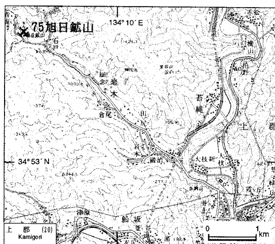
第43図. 旭日鉱山の位置図. 国土地理院発行5万分の1地形図「上郡」を使用.
