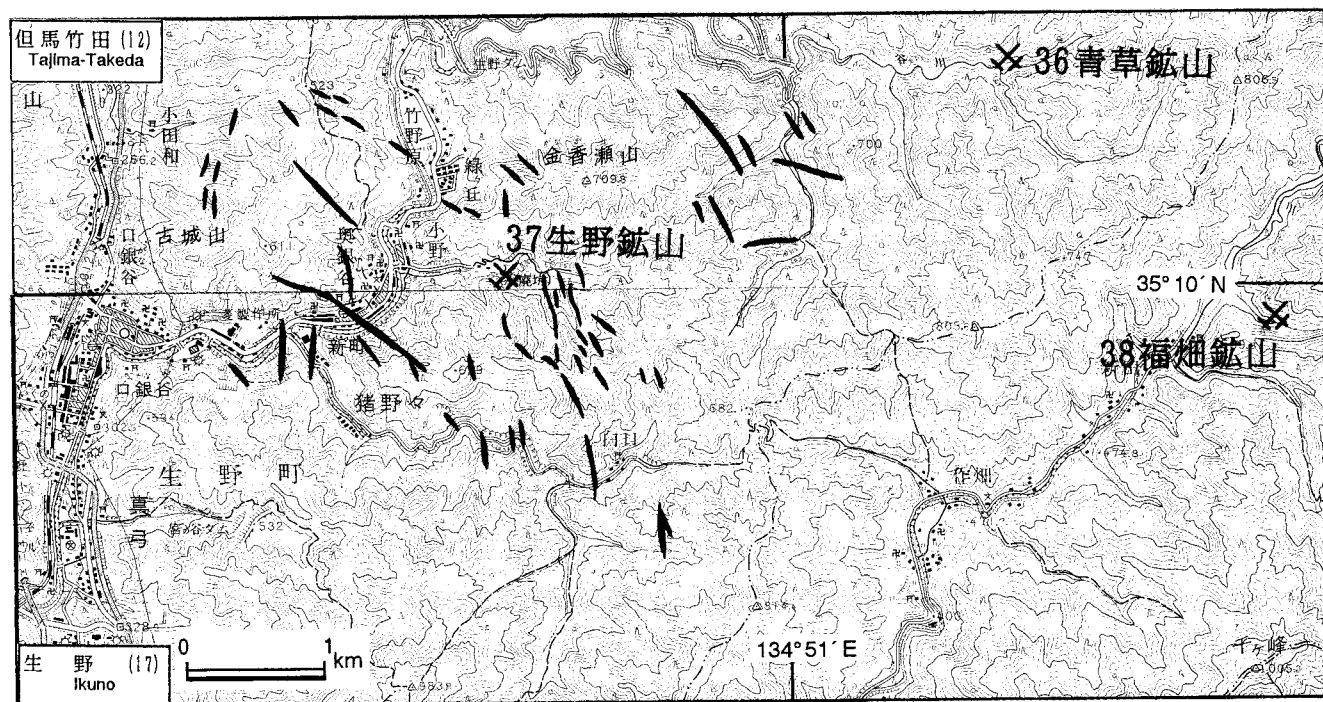
第15図. 青草鉱山・生野鉱山・福畑鉱山の位置図. 国土地理院発行5万分の1地形図「但馬竹田」「生野」を使用。
