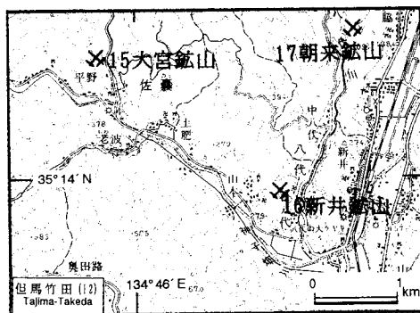
第8図. 大宮鉾山・新井鉾山・朝来鉾山の位置図。国土地理院発行5万分の1地理図「但馬竹田」を使用。
