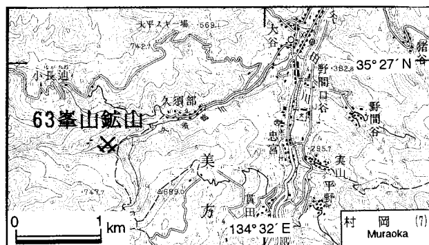
第32図. 峯山鉱山の位置図。国土地理院発行5万分の1地形図「村岡」を使用。
