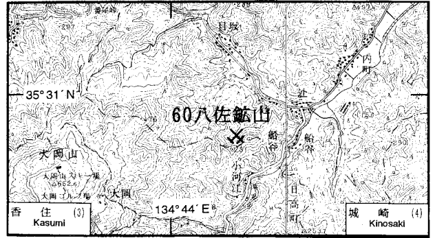
第29図. 八佐鉱山の位置図. 国土地理院発行5万分の1地形図「香住」「城崎」を使用.
