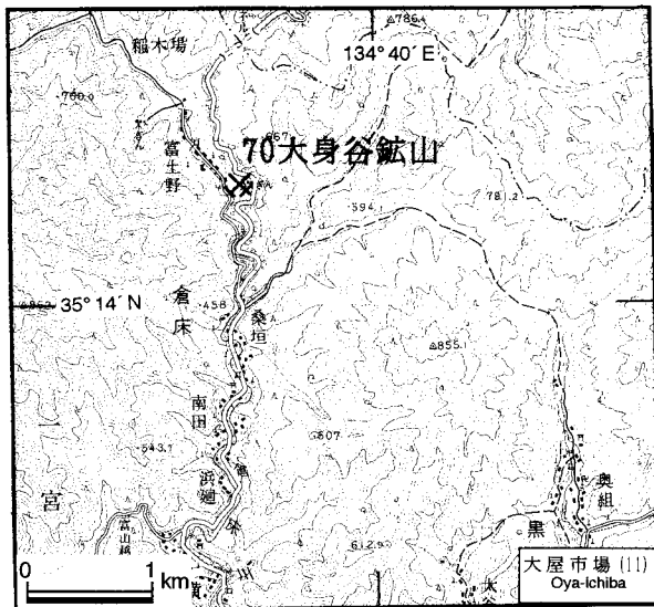
第38図. 大身谷鉱山の位置図. 国土地理院発行5万分の1地形図「大屋市場」を使用.
