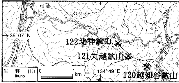
第70図. 越知谷鉱山・丸越鉱山・北神鉱山の位置図. 国土地理院発行5万分の1地形図「生野」を使用.
