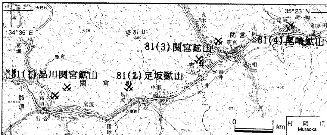
第49図. 品川関宮鉱山・足坂鉱山・関宮鉱山・尾崎鉱山の位置図. 国土地理院発行5万分の1地形図「村岡」を使用.
