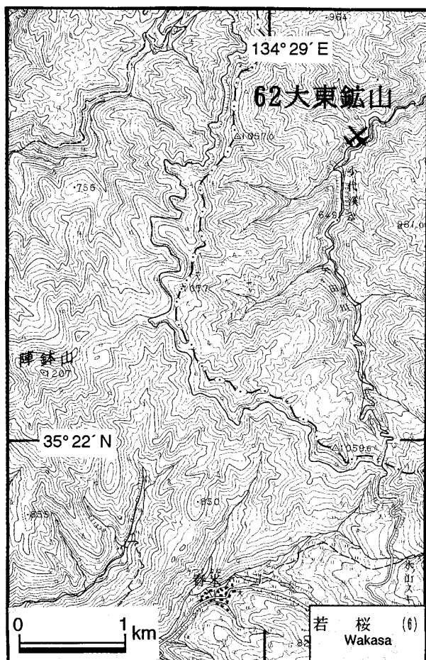
第31図. 大東鉱山の位置図。国土地理院発行5万分の1地形図「若桜」を使用。
