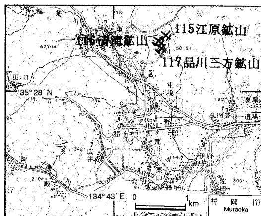
第68図. 江原鉱山・清滝鉱山・品川三方鉱山の位置図. 国土地理院発行5万分の1地形図「村岡」を使用.
