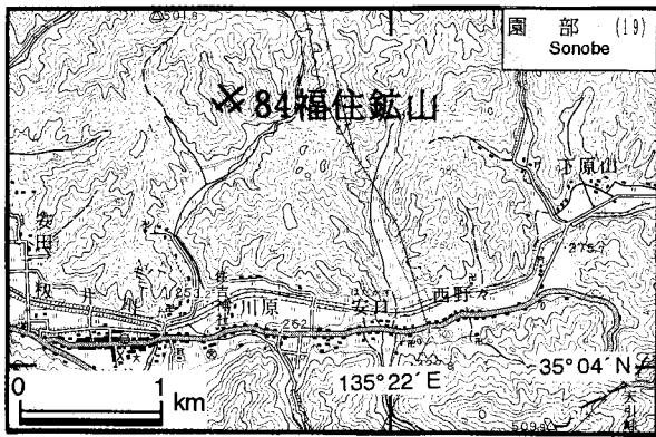
第52図. 福住鉱山の位置図. 国土地理院発行5万分の1地形図「園部」を使用.
