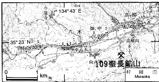
第62図. 聖長鉱山の位置図。国土地理院発行5万分の1地形図「村岡」を使用。
