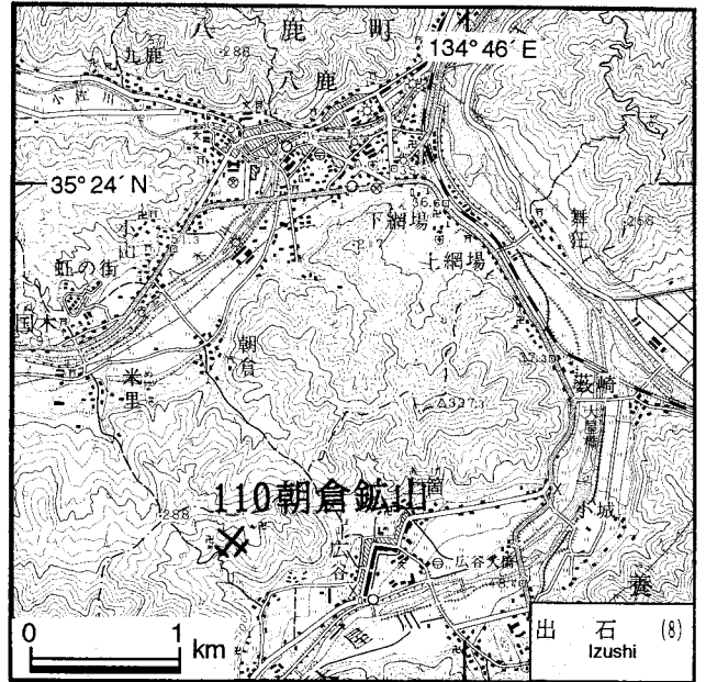
第63図. 朝倉鉱山の位置図。国土地理院発行5万分の1地形図「出石」を使用。
