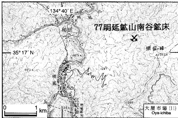
第46図. 明延鉱山南谷鉱床の位置図. 国土地理院発行5万分の1地形図「大屋市場」を使用.
