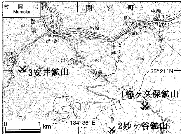
第2図 梅ヶ久保鉱山・妙ヶ谷鉱山・安井鉱山の位置図。国土地理院発行5万分の1地形図「村岡」を使用。
