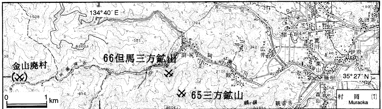
第34図. 三方鉱山・但馬三方鉱山の位置図。国土地理院発行5万分の1地形図「村岡」を使用。
