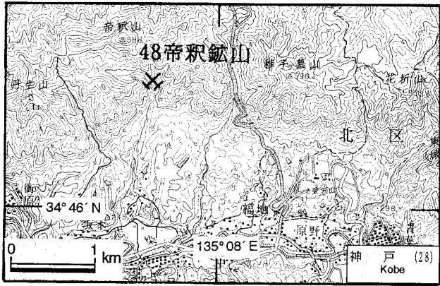
第22図. 帝釈鉱山の位置図. 国土地理院発行5万分の1地形図「神戸」を使用.
