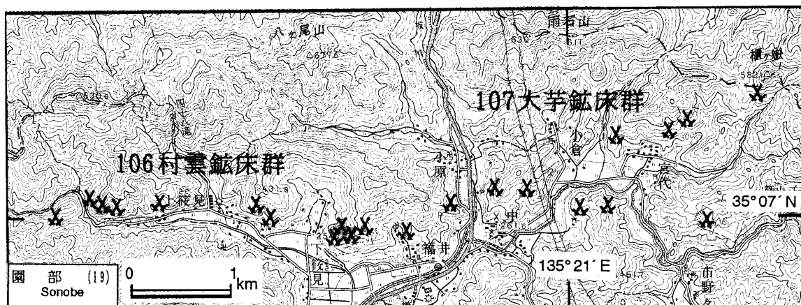
第60図. 村雲鉱床群, 大芋鉱床群の位置図. 国土地理院発行5万分の1地形図「園部」を使用.
