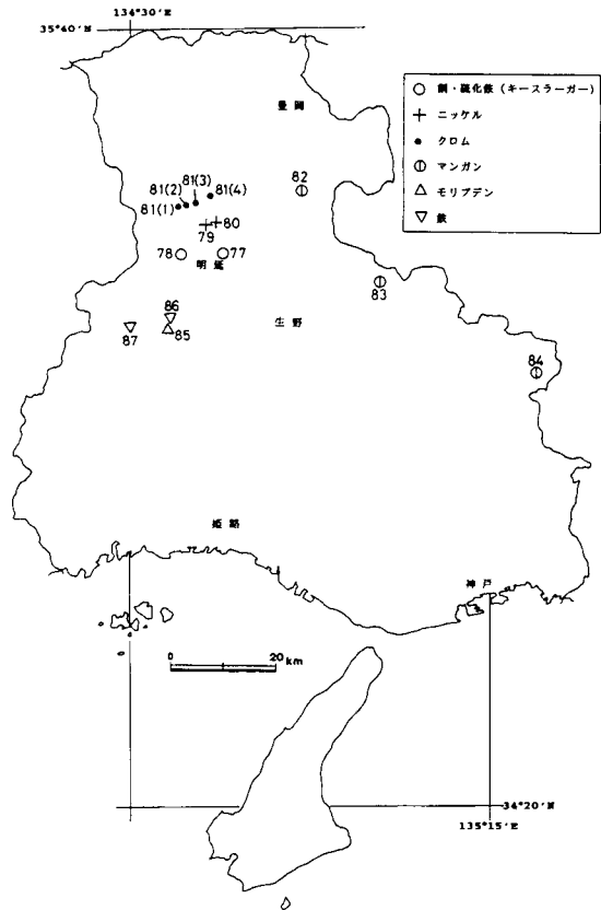
第45図. 兵庫県下の銅・硫化鉄鉱床, ニッケル鉱床, クロム鉱床, マンガン鉱床, モリブデン鉱床, 鉄鉱床の分布, 番号は本文中の鉱山・鉱床の番号に対応する。
