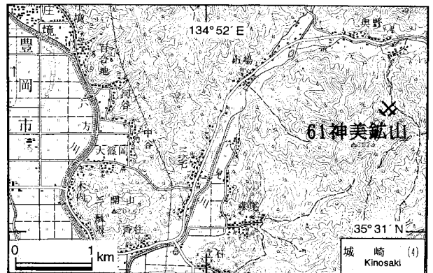
第30図. 神美鉱山の位置図. 国土地理院発行5万分の1地形図「城崎」を使用.
